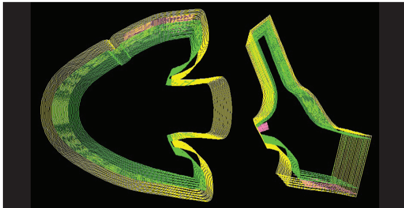
Jedna z funkcií grafického systému je automatické stupňovanie dielcov do celého veľkostného sortimentu
